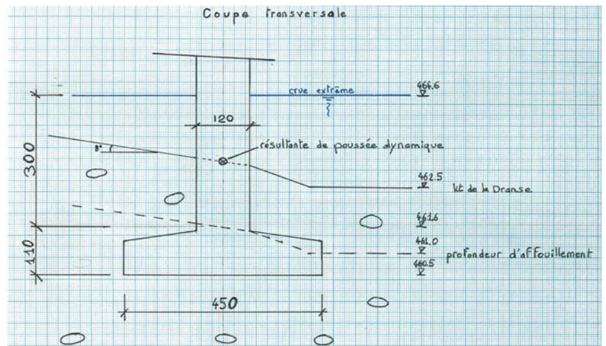
Coupe de la fondation de la pile rive gauche du Pont sur la Dranse
