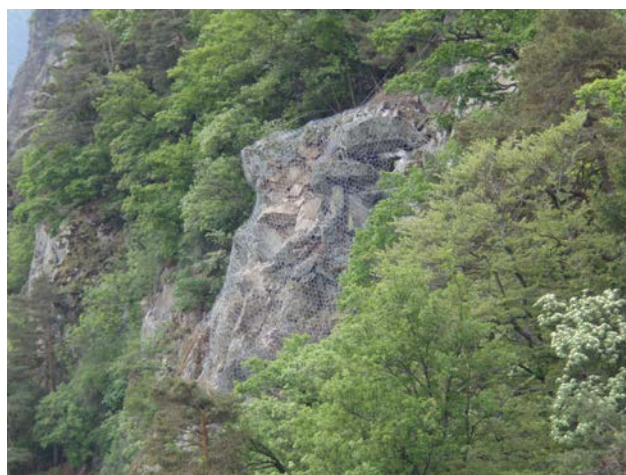
Pose de 560 m 2 de filet couvrant à anneaux sur l'aléa responsable de la chute de blocs du 7.12.2010."
